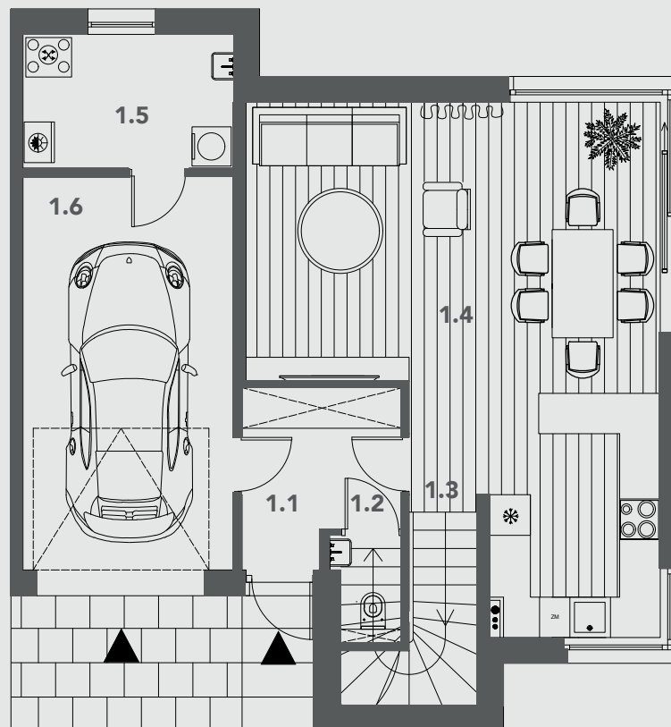
Rzut Parteru
